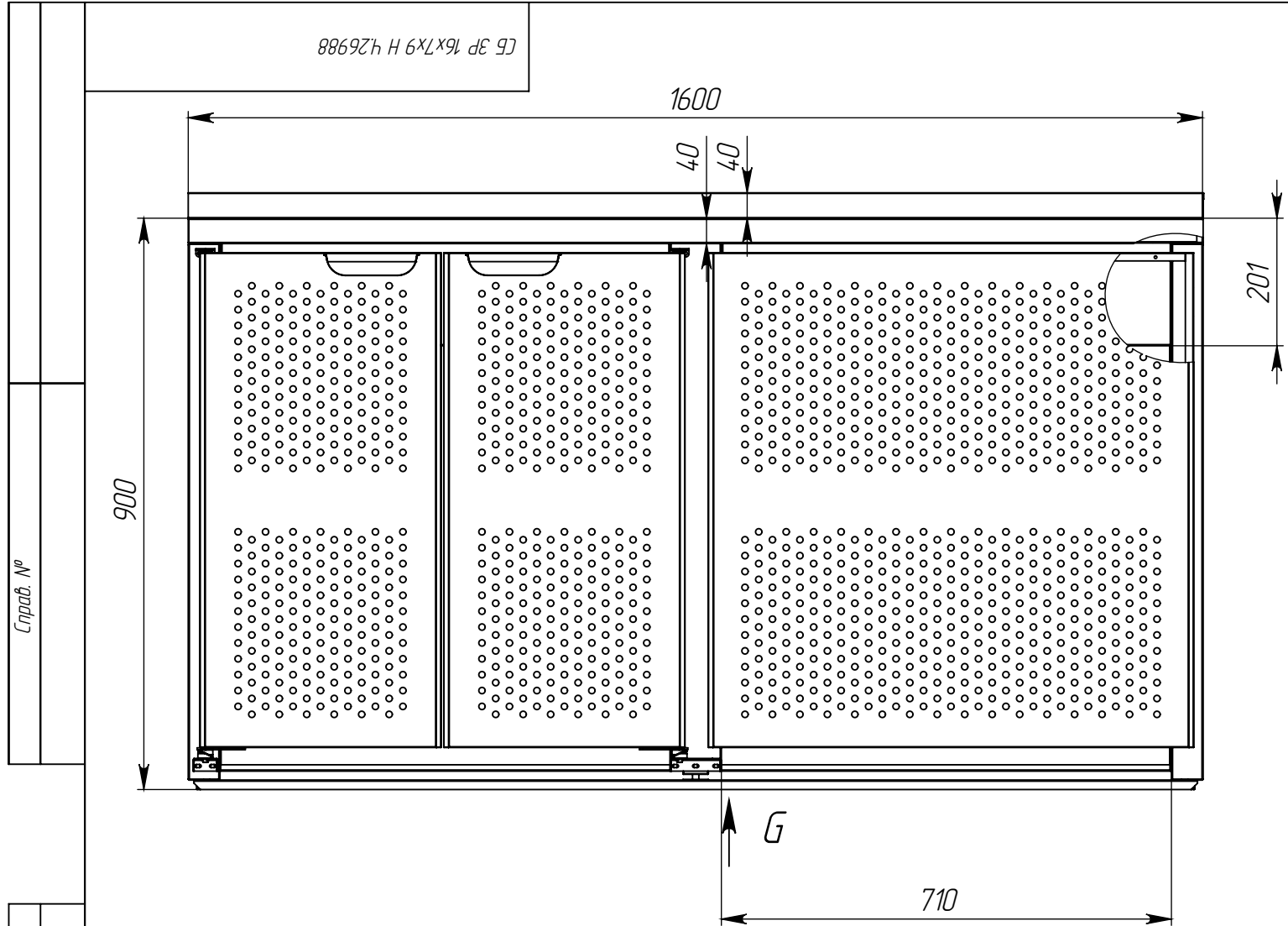
ВИД G
